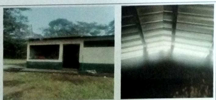
Foto 6: MODULO COCINA ANEXO A MODULO SERVICIO SANITARIO. Cambio de estructura de metal en mal estado por estructura de metal a base de costaneras. Cambio de lamina de zinc por lamina troquelada cal 26.
