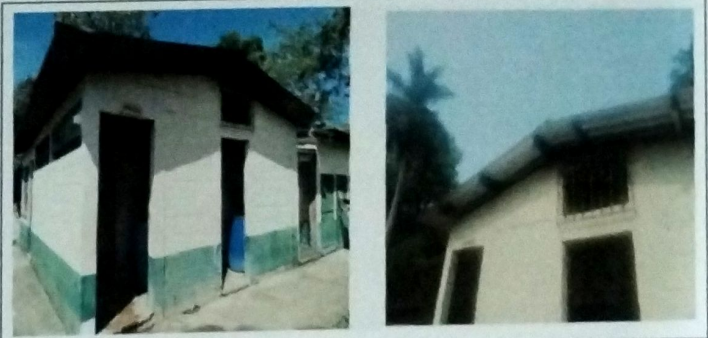
Foto 2: VISTA MODULO D SERVICIOS SANITARIOS. Cambio de estructura de metal en mal estado por estructura de metal a base de costaneras. Cambio de lamina de zinc por lamina troquelada cal 26.
